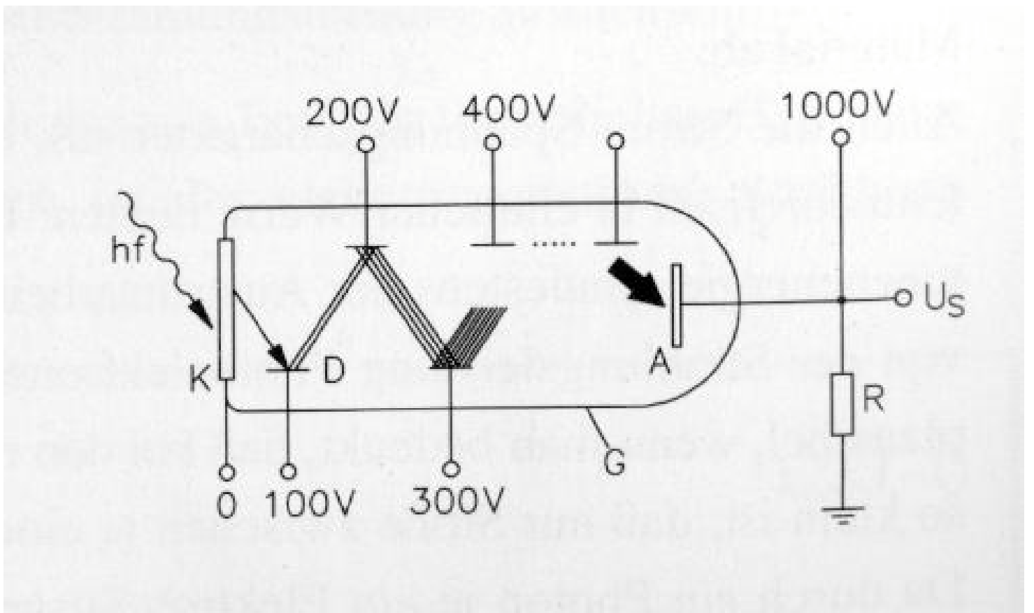
Photoverstärker (Photomultiplier)
