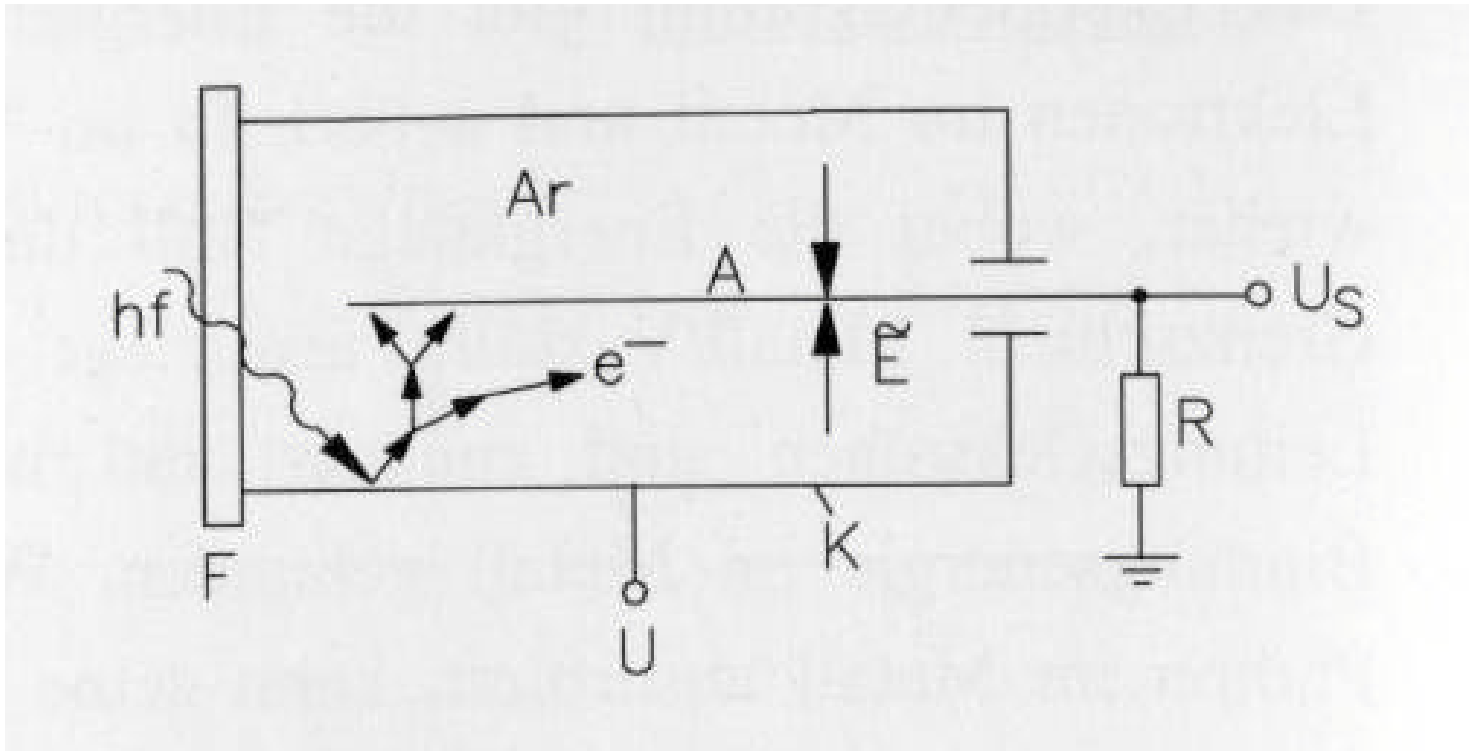
Geigerzähler
