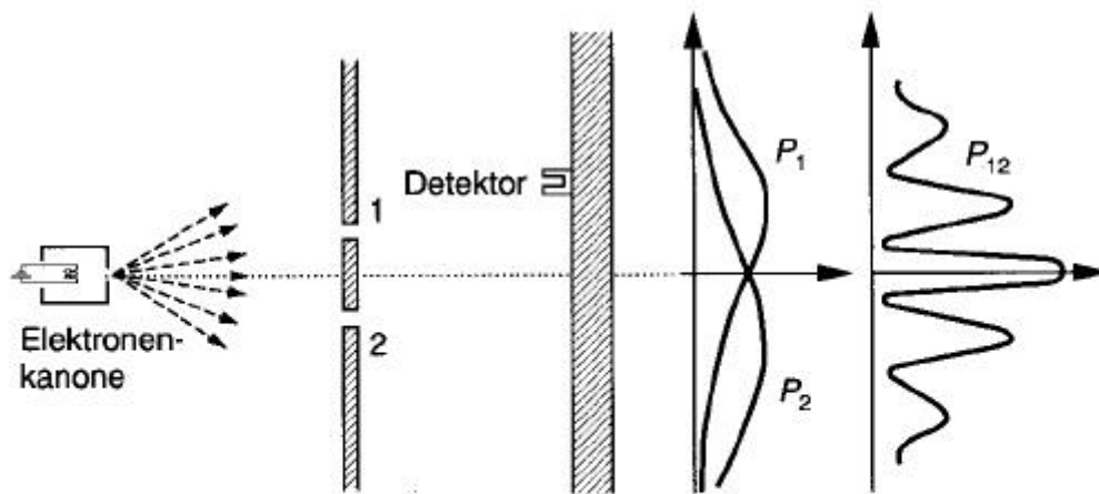
Überlagerung der Verteilungen bei Elektronen
