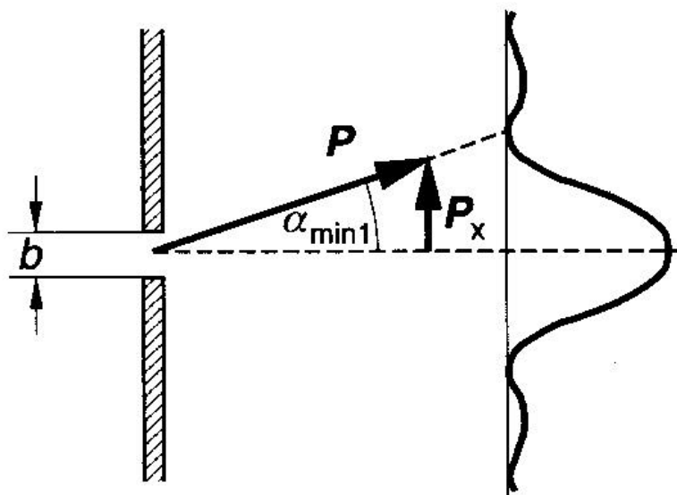
Zur HEISENBERGSchen Unschärfenrelation
