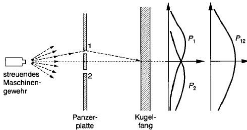
Überlagerung von Verteilungen bei makroskopischen Kugeln
