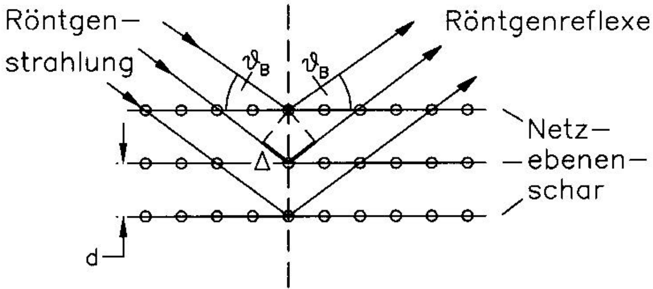
Braggsche Reflexion an Kristallgitter-Netzebenen
