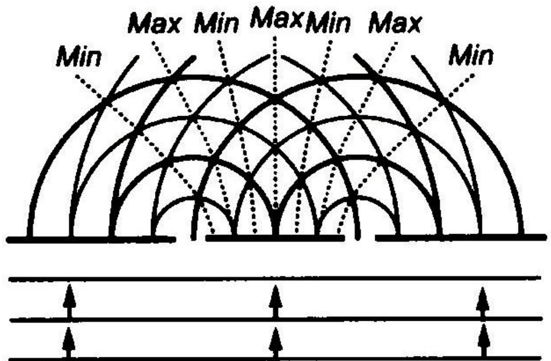
Beugung am Doppelspalt
