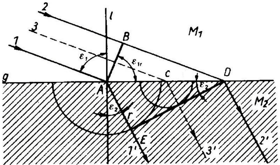
Brechung paralleler Strahlen nach dem Huygensschen Prinzip
